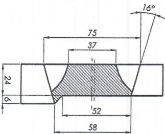
Presjek B-B
