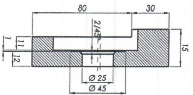
Presjek A-A
